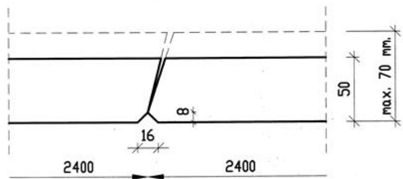
Voegdetail
